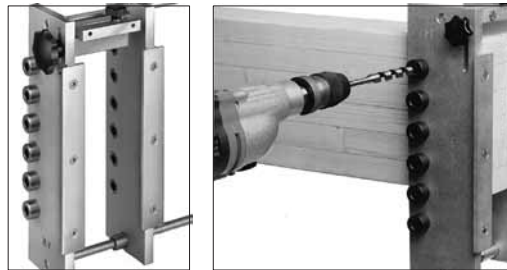
Joist and support bracket / skrytá papuča trámu
