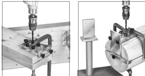
for/pre: joist and support bracket 90 / skrytá papuča trámu 90
