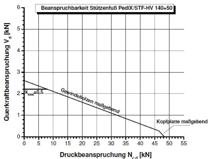
Abbildung B-2: Tragfähigkeiten des Stützenfußes PediX/STF-HV 140+50 bei Interaktion von Druck- und Querkraftbeanspruchungen für angenommene Teilsicherheitsbeiwerte \gamma_M = 1,3 , \gamma_{M0} = 1,0 , \gamma_{M1} = 1,1 und \gamma_{M2} = 1,25
