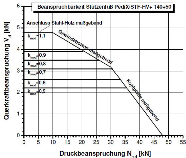
Abbildung B-6: Tragfähigkeiten des Stützenfußes PediX/STF HV+ 140+50 bei Interaktion von Druck- und Querkraftbeanspruchungen für angenommene Teilsicherheitsbeiwerte \gamma_M = 1,3 , \gamma_{M0} = 1,0 , \gamma_{M1} = 1,1 und \gamma_{M2} = 1,25
