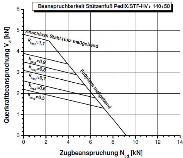
Abbildung B-5: Tragfähigkeiten des Stützenfußes PediX/STF HV+ 140+50 bei Interaktion von Zug- und Querkraftbeanspruchungen für angenommene Teilsicherheitsbeiwerte \gamma_M = 1,3 , \gamma_{M0} = 1,0 , \gamma_{M1} = 1,1 und \gamma_{M2} = 1,25
