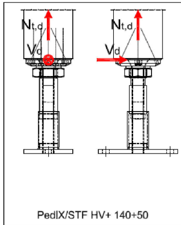
Abbildung B-6: Tragfähigkeiten des Stützenfußes PediX/STF HV+ 140+50 bei Interaktion von Druck- und Querkraftbeanspruchungen für angenommene Teilsicherheitsbeiwerte \gamma_M = 1,3 , \gamma_{M0} = 1,0 , \gamma_{M1} = 1,1 und \gamma_{M2} = 1,25
