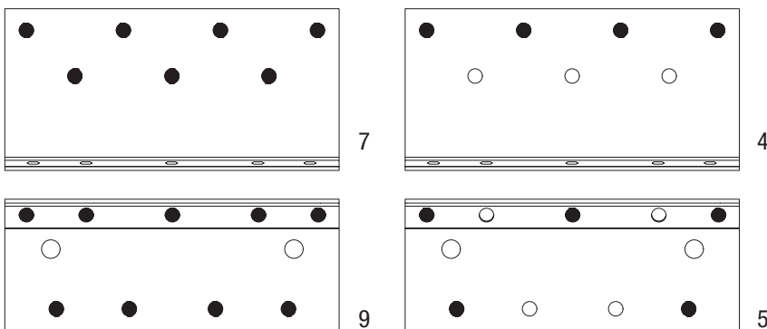
Schraubbild 1
