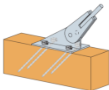
Windverbandschluss mit ZYKT
