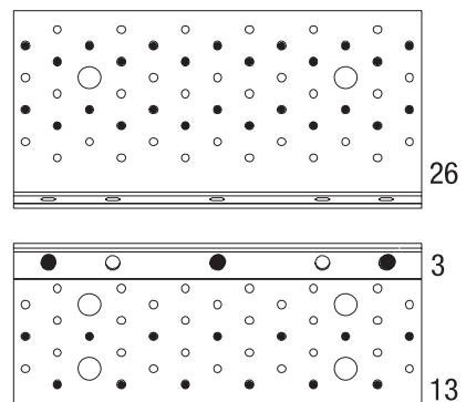
Nagelbild 3
