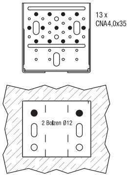
Nagel-/Bolzenbild: A
