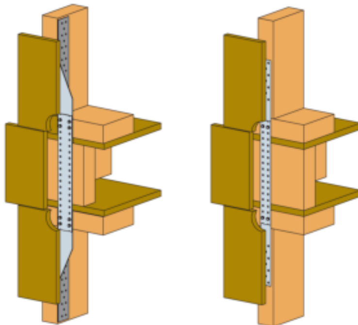
SCMF55/HDUL/R380 in der Anwendung
