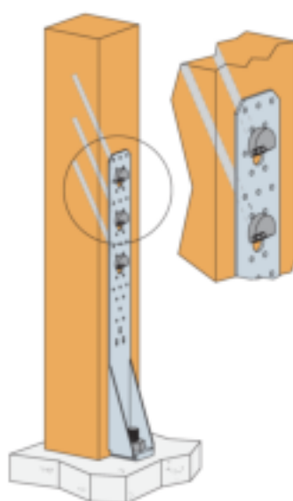
HTT22E Zuganker mit ZYKT
