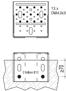
Nagel-/Bolzenbild: C
