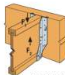
Anschluss Stegträger an Vollholz oder Holzwerkstoff.
