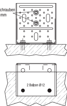
Nagel-/Bolzenbild: E
