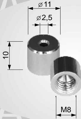
30990-0730 dome nut M8 Hutmutter M8 écrou borgne M8
