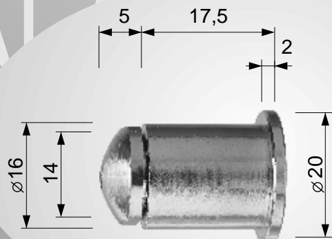
30990-0520 ceiling connector Deckenbefestiger fixation pour plafond
