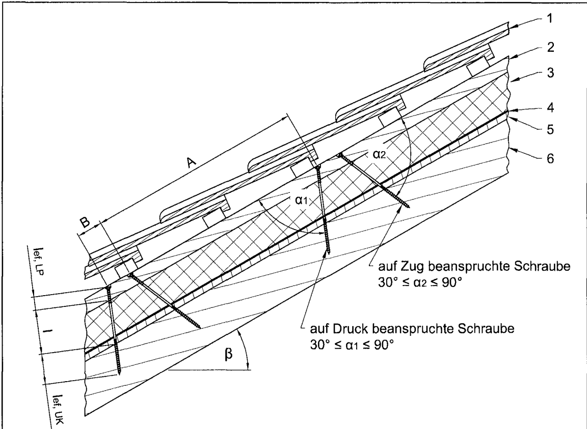
1 - Dacheindeckung, 2 - Konterlatte, 3 - Dämmung, 4 - luftdichte Ebene, 5 - Dachschalung, 6 - Sparren l uf, LP - Gewindelänge in der Konterlatte; l uf, UK - Gewindelänge im Sparren; l - freie Länge der Schrauben
